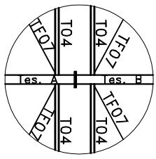
Detalle 01 Lig. tirantes flexíveis com terças
