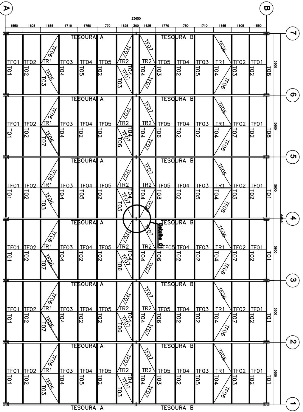
DIAGRAMA DE COBERTURA
